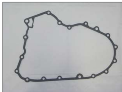
48837 K48900CL CASE ID: BMXA, SLXA 2001 CIVIC OEM #21811-PLX-000
